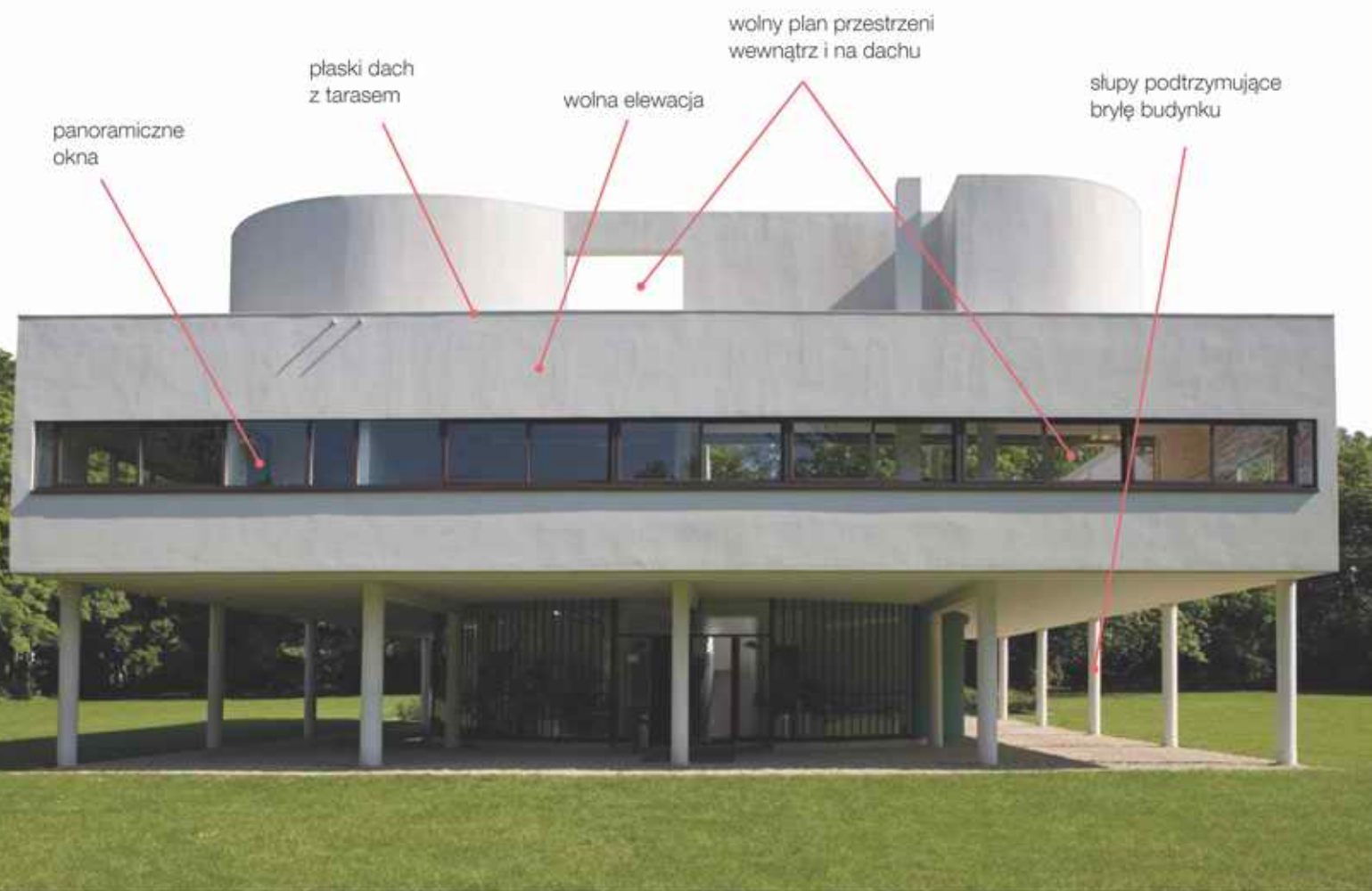
Willa Savoye [sawła] w Poissy [plasi] we Francji, architekt Le Corbusier, 1928–1930
